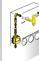
Art. 37830 Kit contaltri digitale per bar olio composto da: - Art. 37780 contaltri digitale - raccordi di collegamento - attacchi M 1/2" x F 1/2" - non omologato per uso pubblico
