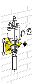
Art. 10/12 Staffa murale in acciaio verniciato per fissaggio a parete di pompe industriali dissociate, serie 900 e 1200
