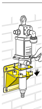
Art. 10/11 Staffa murale in acciaio verniciato con ammortizzatori per fissaggio a parete di pompe industriali integrali e flangiate, serie 900 e 1200
