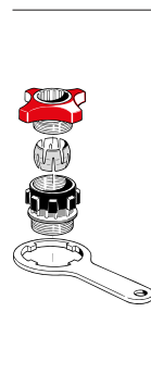
Art. 33434 Ghiera di bloccaggio \varnothing 34 mm, a doppio corpo per pompe con pescante, serie 600 inox
