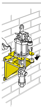
Art. 10/17 Staffa murale in acciaio verniciato con ammortizzatori per fissaggio a parete di pompe industriali flangiate, serie 1500 - 1800
