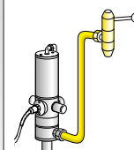
Art. 37683 Rubinetto bar olio con collegamento a pompa, composto da: - Art. 37681 rubinetto bar olio - Art. 37682 tubo di collegamento rubinetto/pompa
