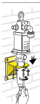
Art. 10/10 Staffa murale in acciaio verniciato per fissaggio a parete di pompe industriali integrali e flangiate, serie 900 e 1200
