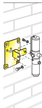
Art. 33115 Staffa murale in acciaio per fissaggio a parete di pompe travaso, serie 600 inox
