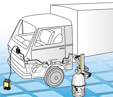
Fase di spurgo di un impianto frizione idraulica
