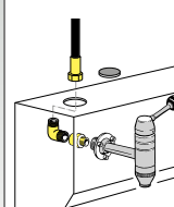
Art. 37693 Kit di collegamento impianto fisso bar olio, composto da: - Art. 996.301 tubo M 1/2" x F 1/2" - 1 m - gomito M 1/2" x M 1/2" - nipple M 1/2" x F 1/2"
