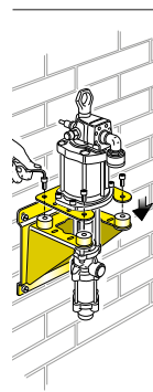
Art. 10/18 Staffa in acciaio verniciato con ammortizzatori per fissaggio a parete di pompe industriali dissociate, con pescante \varnothing 100 mm, serie 900 e 1200
