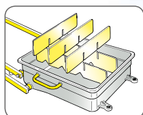
Vasca con frangiflutti
