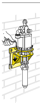
Art. 10/13 Staffa murale in acciaio verniciato con ammortizzatori per fissaggio a parete di pompe industriali dissociate, serie 900 e 1200
