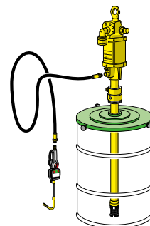
Coprifusto con filetto 2" F per ricevere la ghiera di montaggio pompe
